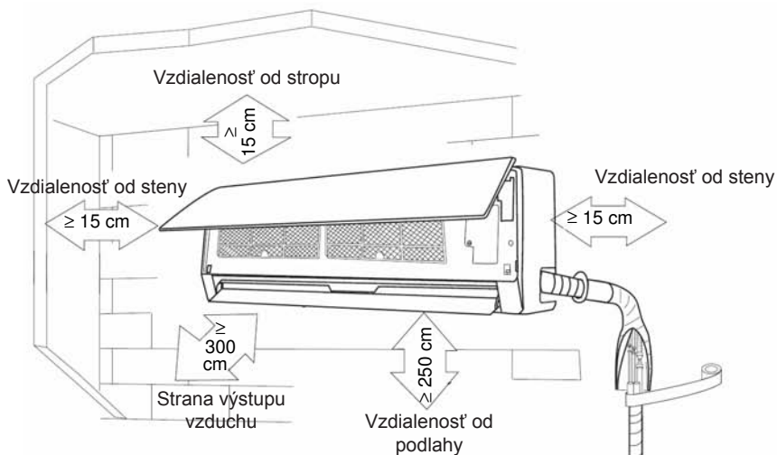
Rozmerový výkres inštalácie
